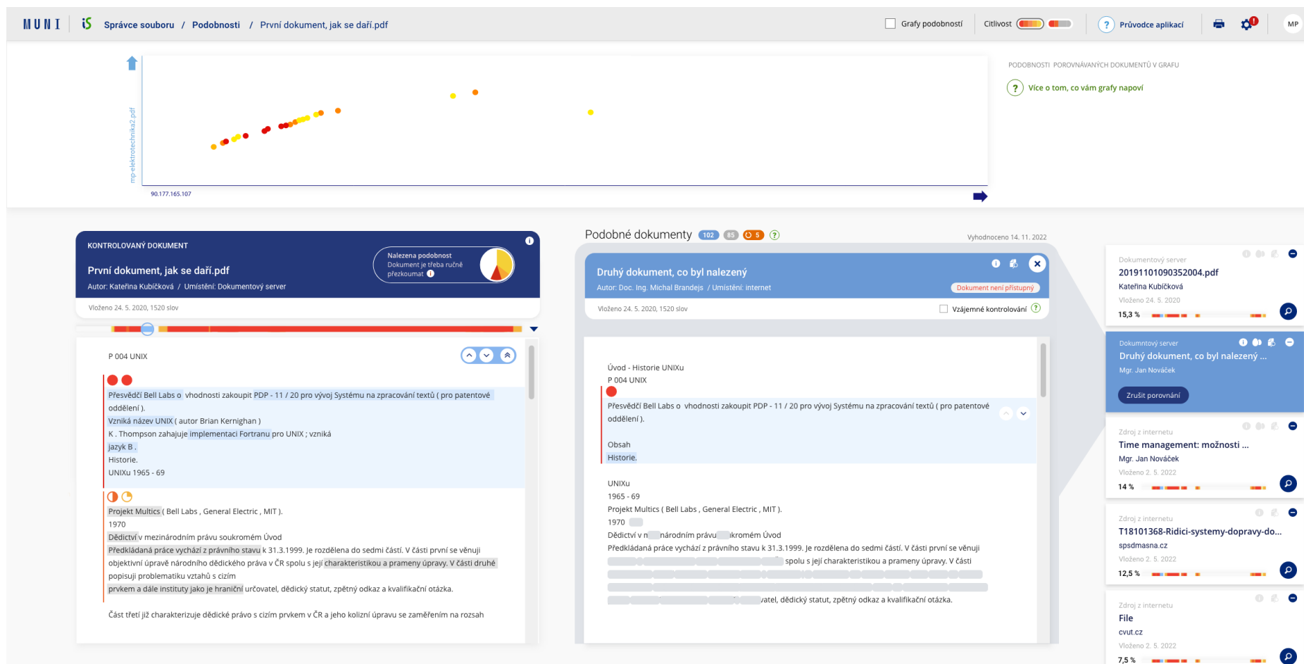
Obr. 4: Porovnání s podobným dokumentem vč. 2D grafu, který ukazuje umístění podobných pasáží v obou dokumentech.
