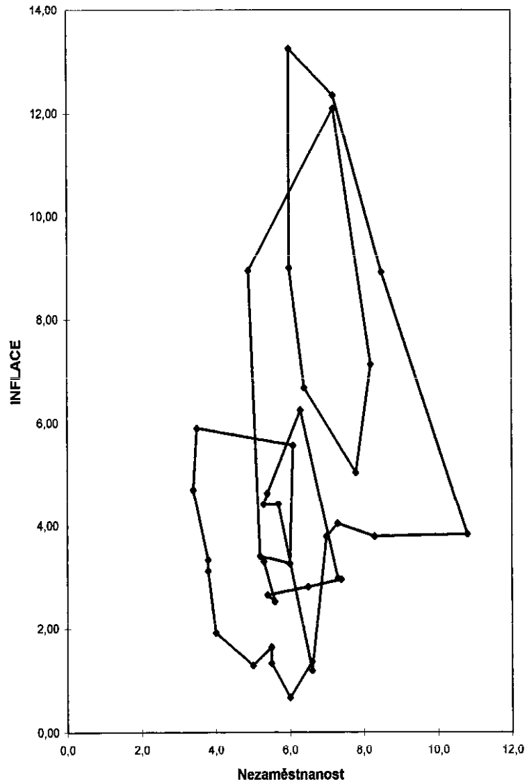
Phillipsova křivka 1960 - 1996
