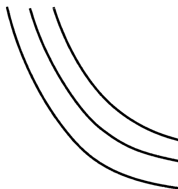
Obr. 20: Izokvanty pro alternativní objemy výroby
