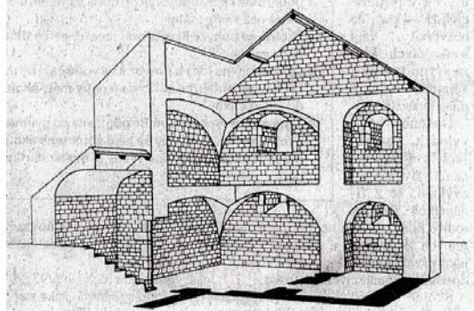
Prostorová rekonstrukce domu čp. 145-146/I - Karlova ulice
