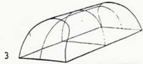
Renesanční klenby: 1 – lunety a výseče vznikají kolmým průnikem dvou valených kleneb; pod tím v půdoryse pár výsečí, křížová klenba a střídavě řazené výseče; 2 – koutové výseče (lunety) v neckové klenbě a jejich půdorys; 3 – necková klenba
