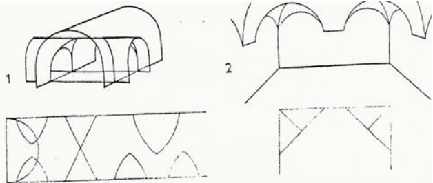
Renesanční klenby: 1 – lunety a výseče vznikají kolmým průnikem dvou valených kleneb; pod tím v půdoryse pár výsečí, křížová klenba a střídavě řazené výseče; 2 – koutové výseče (lunety) v neckové klenbě a jejich půdorys; 3 – necková klenba
