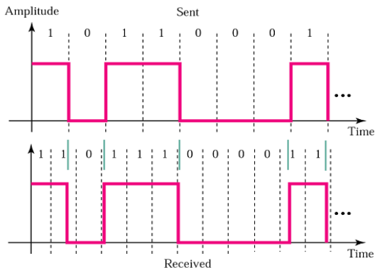
Figure: Ilustrace problému synchronizace vysílače a přijímače (zcela bez synchronizace) – vysílač vysílá 10110001, přijímač přijímá 110111000011.
