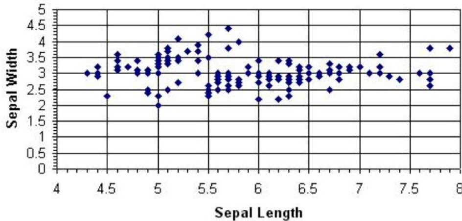
Iris Data
