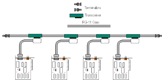
10Base5 Ethernet – schéma zapojení Zdroj: http://physinfo.ulb.ac.be
