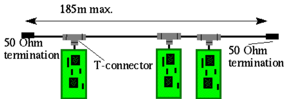
10Base2 Ethernet – schéma zapojení Zdroj: http://www.linuxfocus.org/
