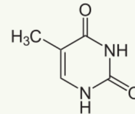
Tymin
