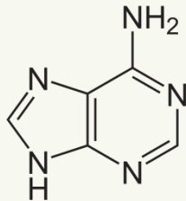
Adenin
