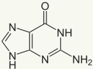
Guanin
