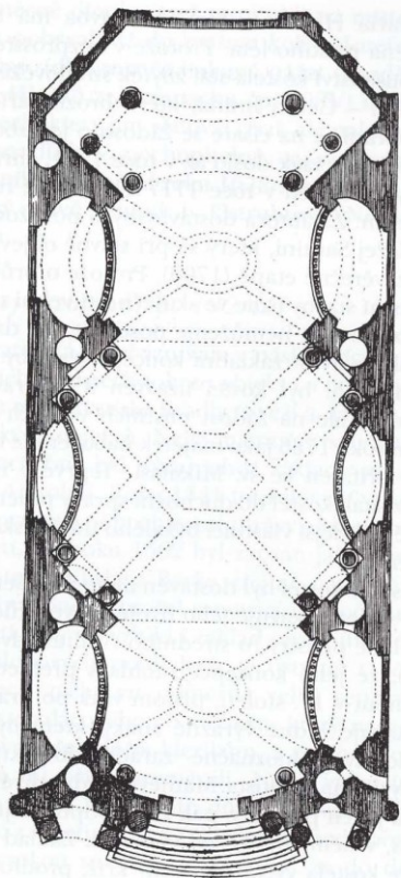
Půdorys podle Guariniho návrhu kostela P. Marie Altoetingské v Praze z roku 1679
