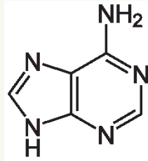
Adenin
