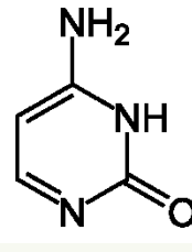
Cytosin
