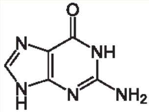
Guanin
