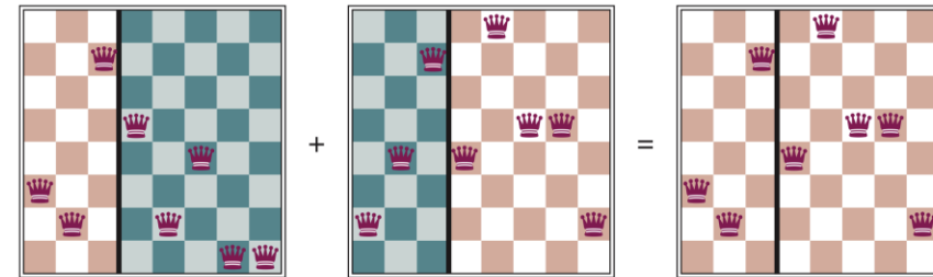
Kombinace prvních dvou řádků odpovídající kroku řešení problému 8 dam na šachovnici
