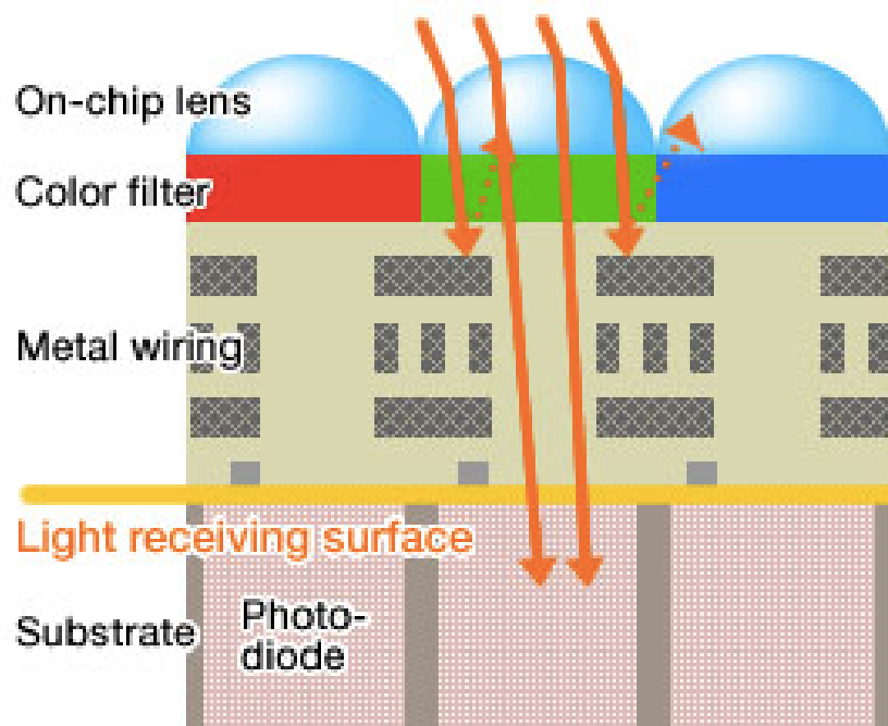
Front-illuminated structure
