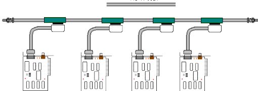
10Base5 Ethernet – schéma zapojení Zdroj: http://physinfo.ulb.ac.be
