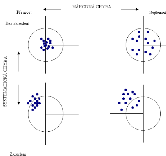
Obr. 3 Znázornění náhodné a systematické chyby
