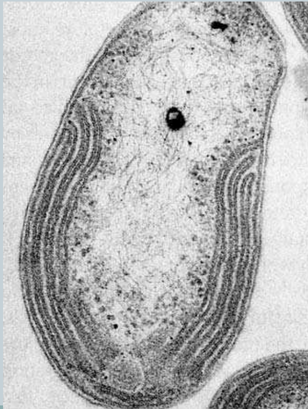
aerobní prokaryota
