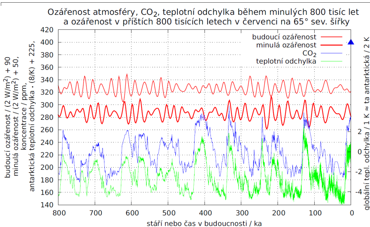
Obrázek 2.2: Červené křivky udávají proměny intenzity ozáření (aneb ozáření) vodorovné plochy ovzduší poblíž polárního kruhu v červenci. Tlustě jsou vyznačeny hodnoty minulé, tenké budoucí. Koncentrace oxidu uhličitého i teplotní anomálie jsou zjištěny z ledových vrtných jader v Antarktidě; antarktická teplotní odchylka jsou zhruba dvojnásobkem anomálií globálních. (Laskar et al. 2004) (Jouzel et al. 2007) (Lüthi et al. 2008). Koncentrace CO 2 v r. 2015, 400 ppm, je vyznačena modrým trojúhelníkem. Zdrojový skript je 800-800ka_cz65.gnp v adresáři amper.ped.muni.cz/gw/aktivita/grafy/sources/ , kde jsou i zdrojová data. Online výpočet viz web “Computation of Various Insolation Quantities for Earth” 2013. (K popiskům: „ka“ je tisíc let, „a“ je značka pro rok z latinského annus ; změnil-li se antarktická teplota o dva kelviny, globální se změní jen o jeden kelvin)
