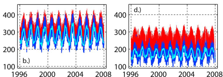
Obrázek 2.1: Sálání oblohy na zem na dvou švýcarských stanicích, Payerne (b., 490 m nad mořem) a Jungfrauoch (d., 3580 m n.m.). Svislá osa udává ozáření ve wattech na metr čtvereční, vodorovná letopočet. Jde o data po 10 min, tmavě modře jen pro chvíle bezoblačné oblohy, červeně pro všechna měření; je zřejmé, že oblačnost k sálání na zem velmi přispívá zejména na vrcholu Jungfrauoch, kde má vzduch velmi nízký obsah vodní páry. Světle modrá křivka ukazuje střední hodnoty pro bezoblačné stavy. Je dobře vidět sezónní cyklus, stanice Payerne je přitom srovnatelná s nížinnými oblastmi Česka. Zdroj: Figure 2 (Wacker et al. 2011). Táž práce dále ukazuje, že se na níže položené stanici sálání z bezoblačné oblohy za ono období zvýšilo nejspíše o 5 \text{ W/m}^2 , vlivem nárůstu teploty a obsahu páry.
