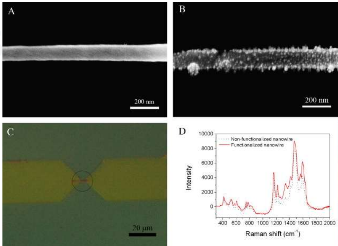
Fig. 1. (A) SEM obraz nemodifikovaného polyanilinového (PANI) nanovlákná (B) SEM obraz modifikovaného PANI nanovlákná IgG protilátkou. (C) Modifikované PANI nanovlákná protilátkou IgG značený fluorescenční sondou Texas Red (v kroužku). (D) Srovnání Ramanova spektra před a po modifikaci PANI nanovlákná
