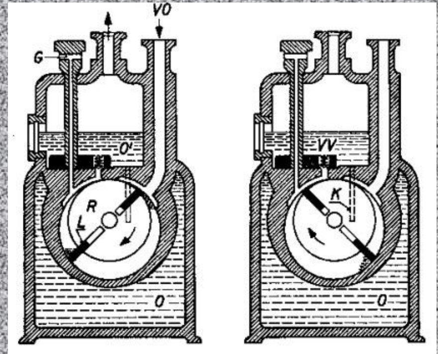
Olejová rotační vývěva
