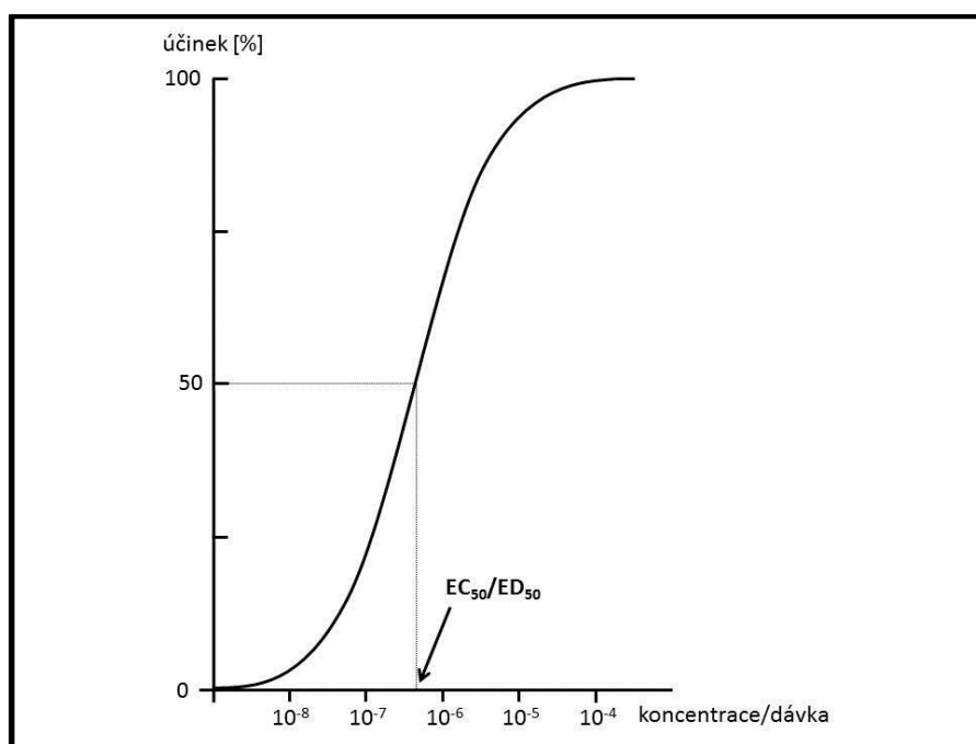
Obr. 7 Vztah dávky a účinku. Typický esovitý tvar křivky závislosti účinku na dávce aplikované látky při semilogaritmickém znázornění (osa x v logaritmickém a osa y v lineárním měřítku). EC 50 a ED 50 vyjadřují koncentraci respektive dávku potřebnou k dosažení 50% maximálního možného efektu.
