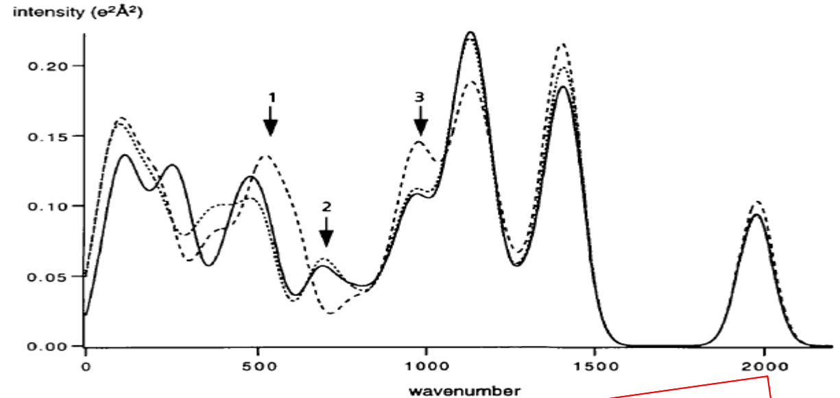
6-undecanone ———
