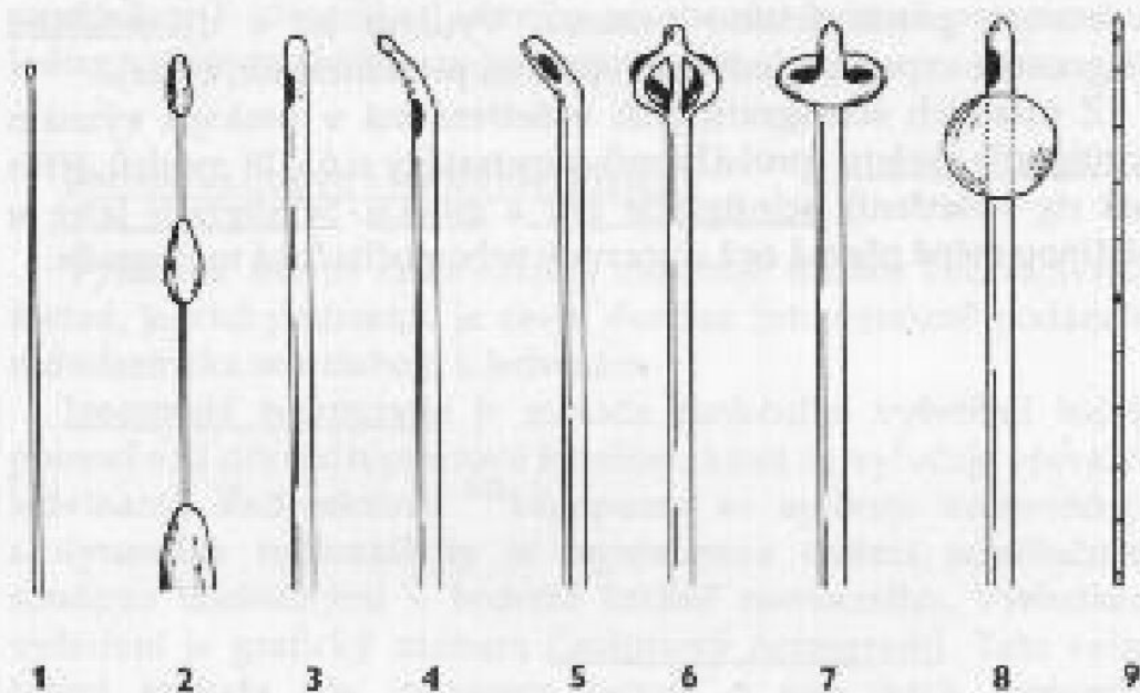
Obr. 13. Základní urologické cévky a sondy: 1 - filiformní sonda, 2 - bužie à boule, 3 - cévka Nelatonova, 4 - Tiemannova, 5 - Mercierova, 6 - Malecotova, 7 - Pezzerova, 8 - balónková, 9 - ureterální
