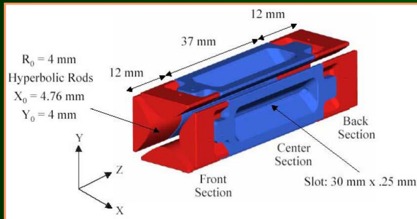
Lineární iontová past
