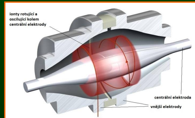
Orbitrap
