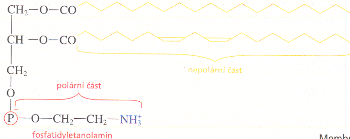
Membránový fosfolipid.
