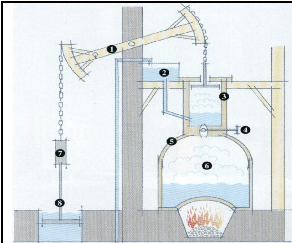
Princip Newcomenova atmosférického parního stroje
