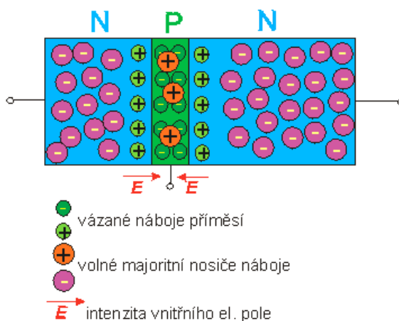
Obr.3.15. Princip činnosti tranzistoru [6].
