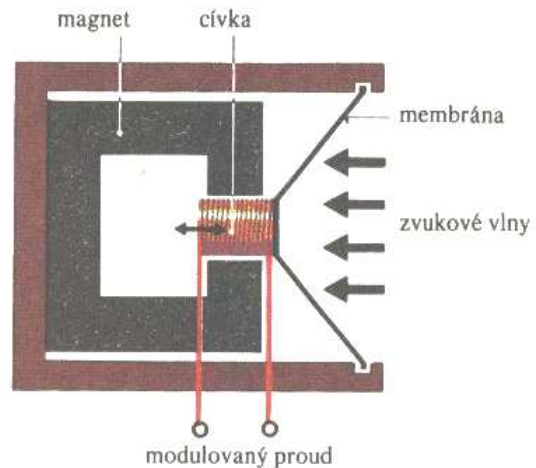
Obr.4.58. Elektromagnetický mikrofon.
