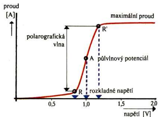
Obr.4.27. Polarografická křivka
