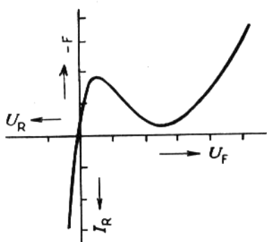
Obr. 3.14. Voltampérová charakteristika tunelové diody.
