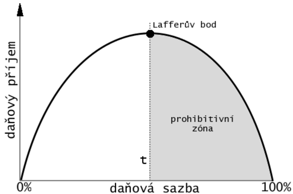
Lafferova křivka
