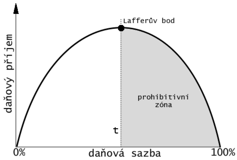
Lafferova křivka
