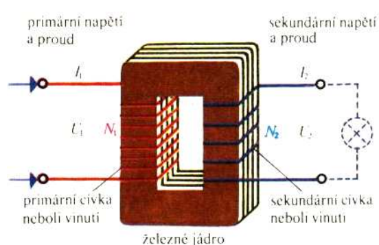
Obr.4.18. Transformátor.
