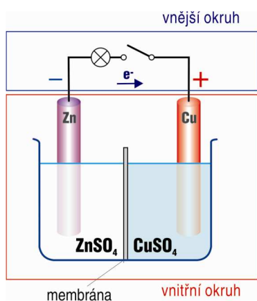
Obr.1.7a) Danielův článek
