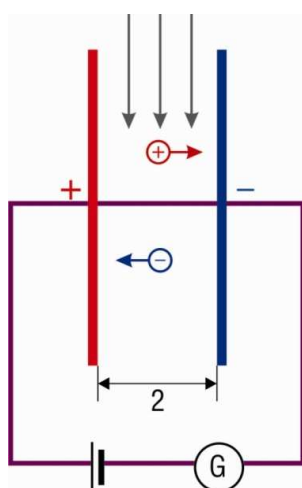
Obr.2.1 a) Schematické znázornění experimentálního uspořádání pro studium vedení elektriny v plynech.
