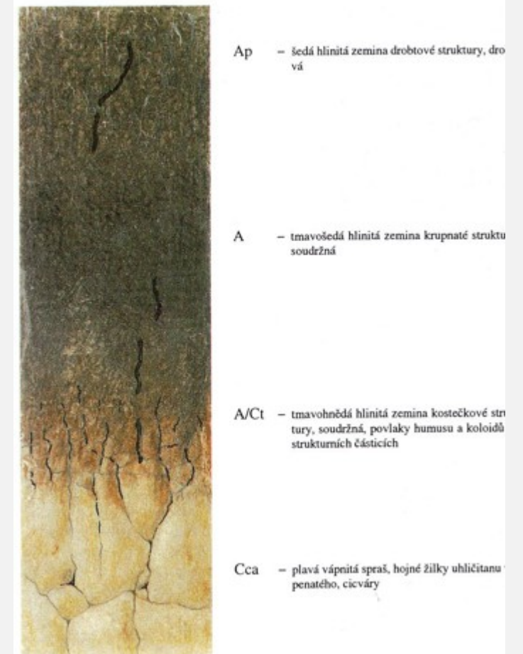
Černozem degradovaná na spraši
