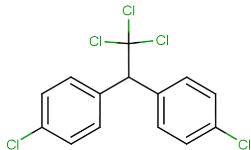
DDT
