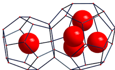
Hydráty (klathráty s ledem)
