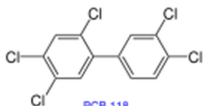
PCB 118
