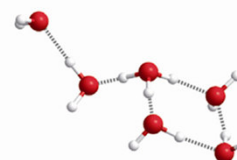
H 3 O + (H 2 O) 5
