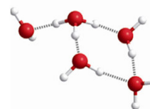
H 3 O + (H 2 O) 4
