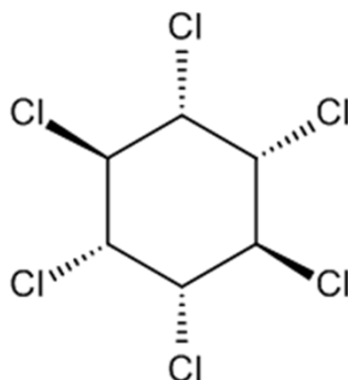
HCH
