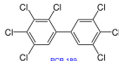
PCB 189
