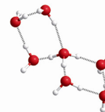
H 3 O + (H 2 O) 6
