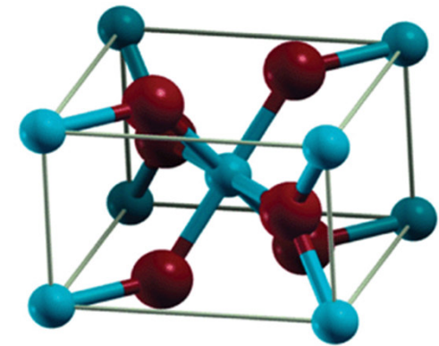
MgH 2
