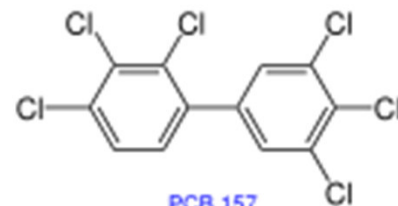
PCB 157
