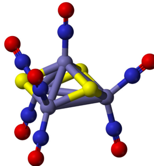
anion Roussinovy černé soli [\text{Fe}_4\text{S}_3(\text{NO})_7]^{-}
