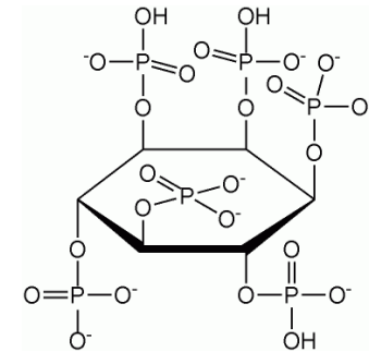
kyselina fytoová
