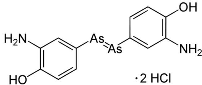
Salvarsan
