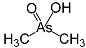
kyselina kakodylová
