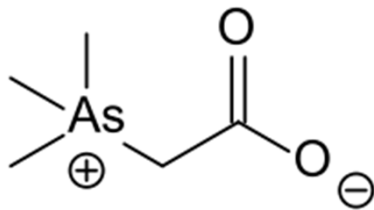
Arsenobetain
