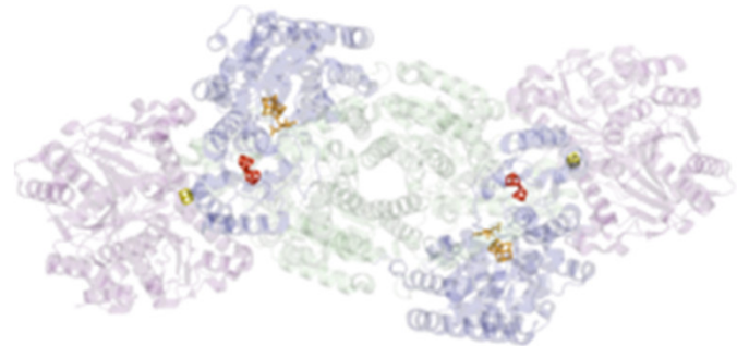
nitrogenáza
