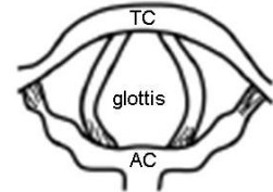
Postavení hlasivek při usilovném dýchání
