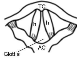
Postavení hlasivek při středně intenzivním dýchání
