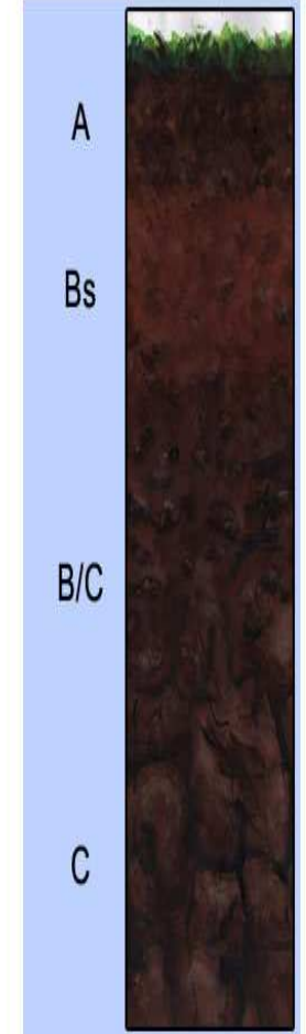
Obr. 8 Kryptopodzol
