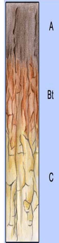
Obr. 7 Hnědozem typická
