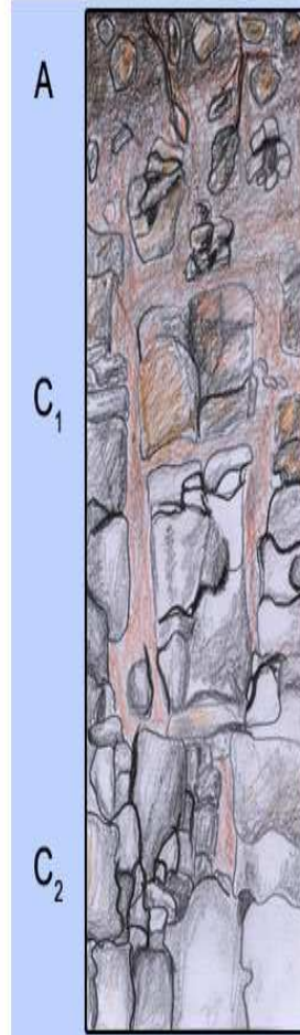
Obr. 2 Rendzina
