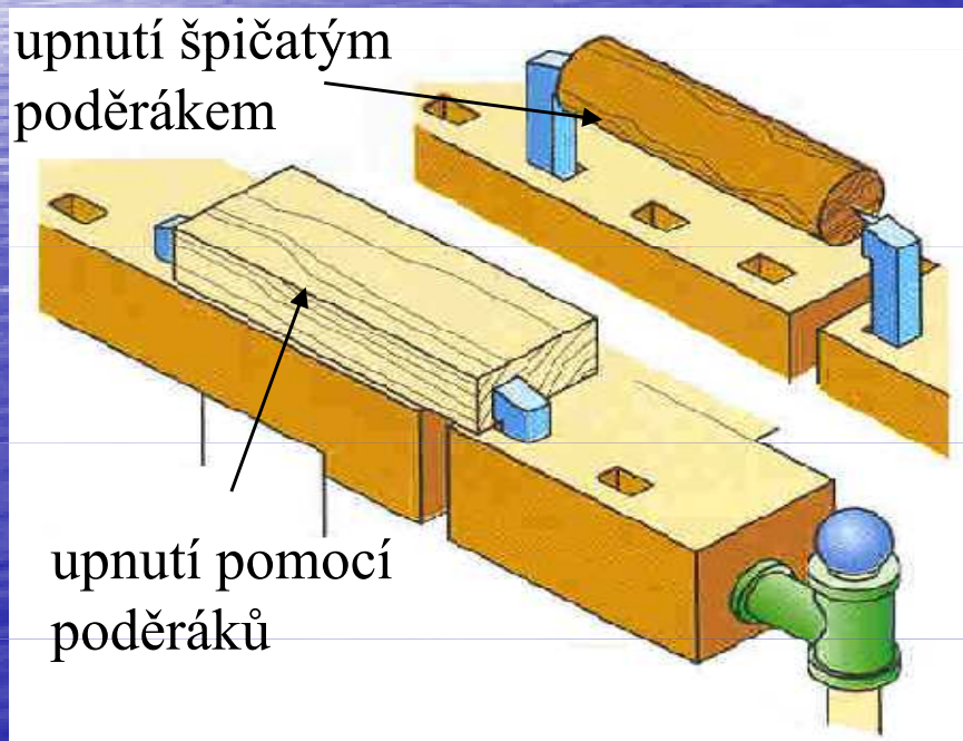
Hoblíce (dražší varianta)
