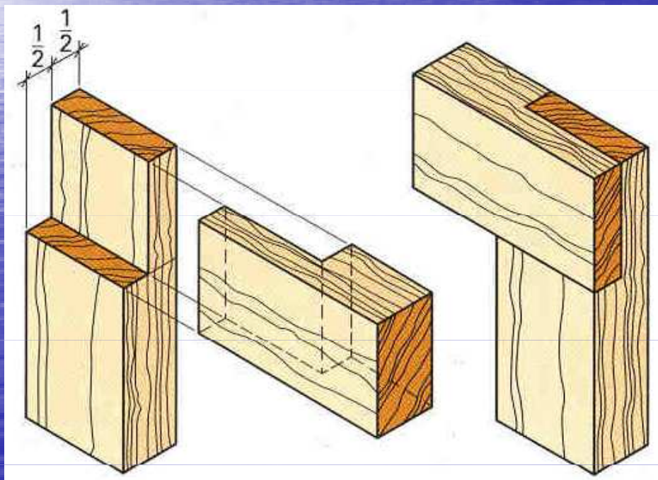
Přeplátování
