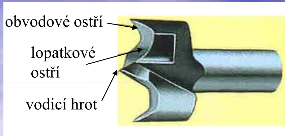
Forstnerův vrták
