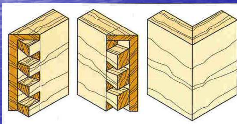
Celokryté ozuby na pokos
