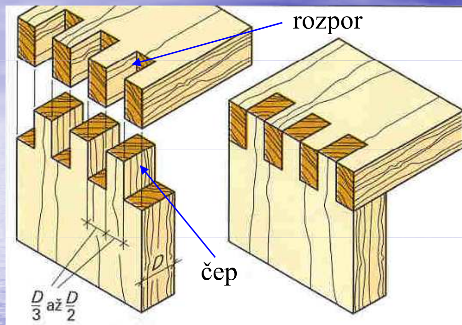
Spoj na sdružené čepy
