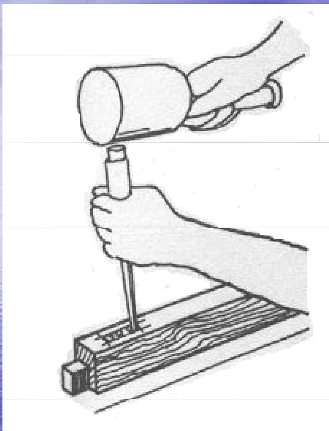
Dlabání s pomocí dřevěné paličky
