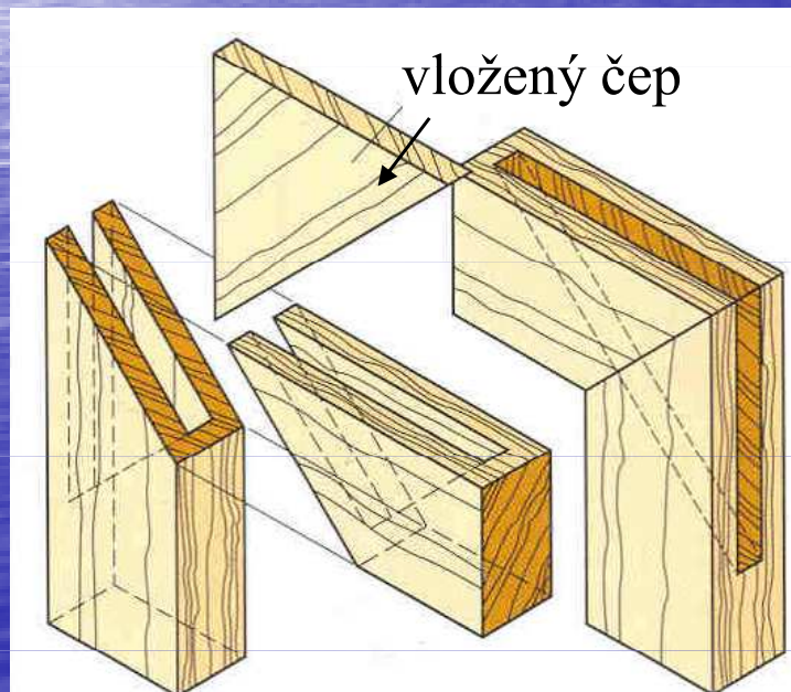
Rohy ráků s vloženým čepem
