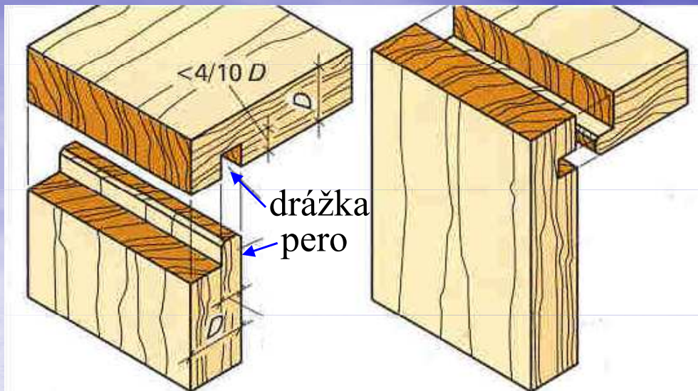
Rohový spoj na péro
