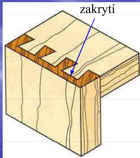
Polokryté spojení ozuby
