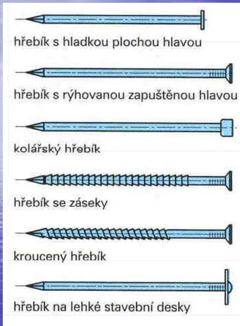
Běžné typy hřebíků
