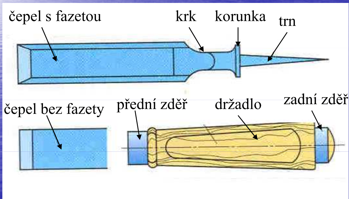
Částí dláta
