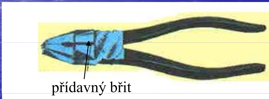
Kombinované kleště
