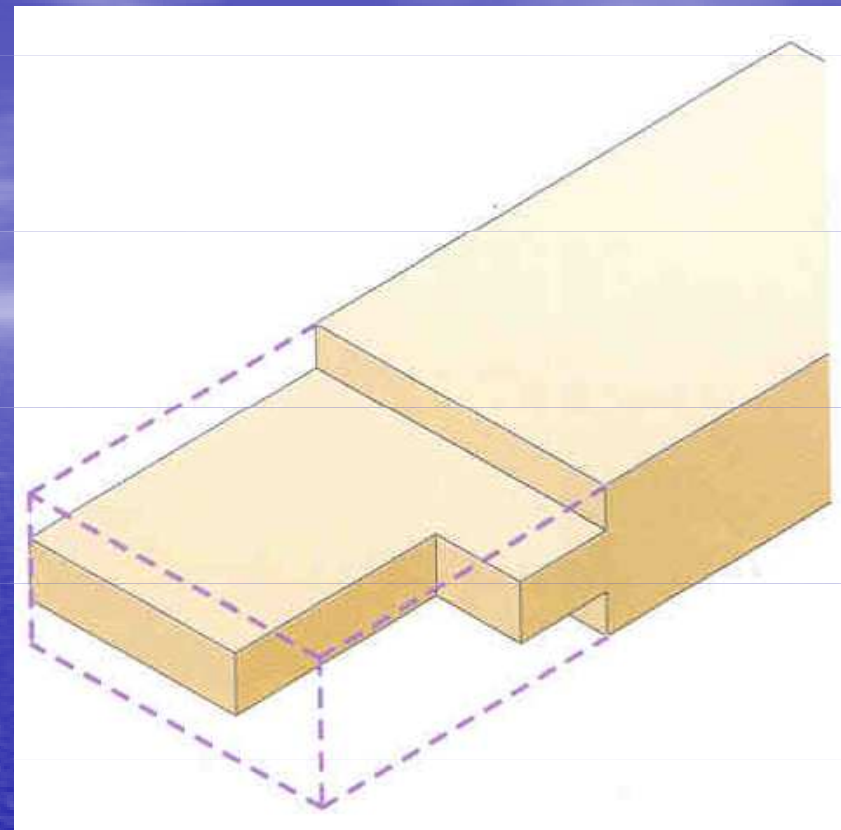
Izometrický náčrt čepu
