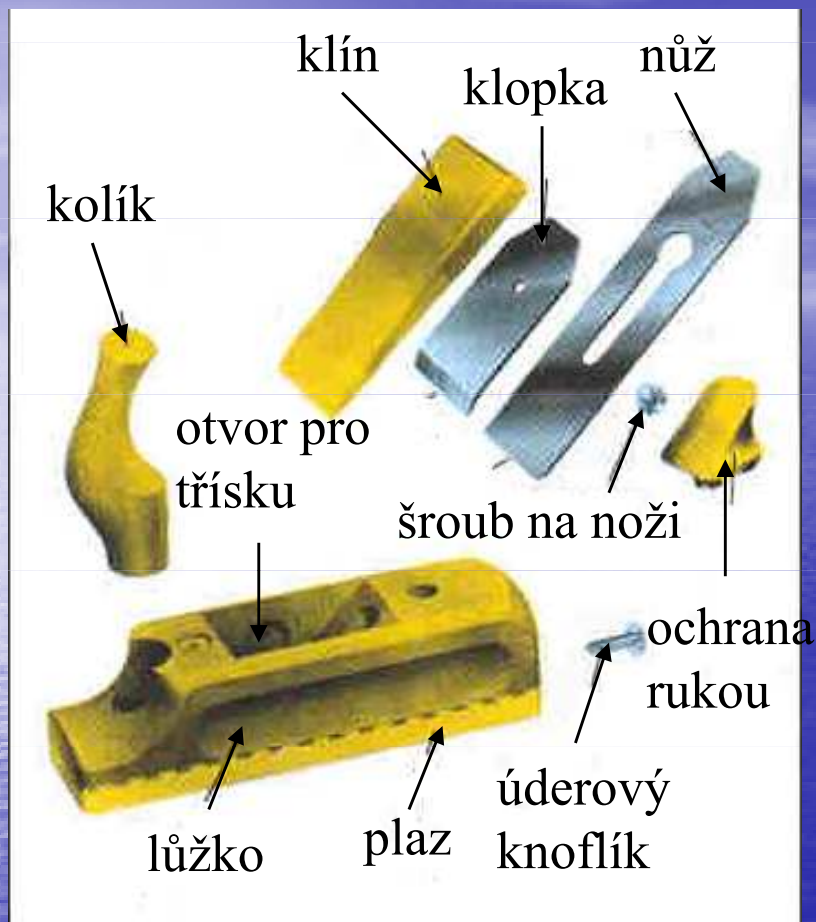
Části hoblíku- klopkaře
