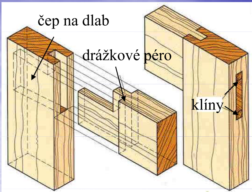
Čep a dlab s pérem
