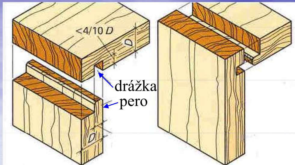
Rohový spoj na péro
