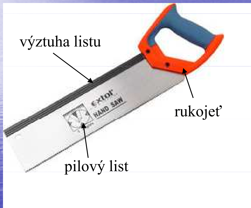
Čepovka s kalenými zuby
