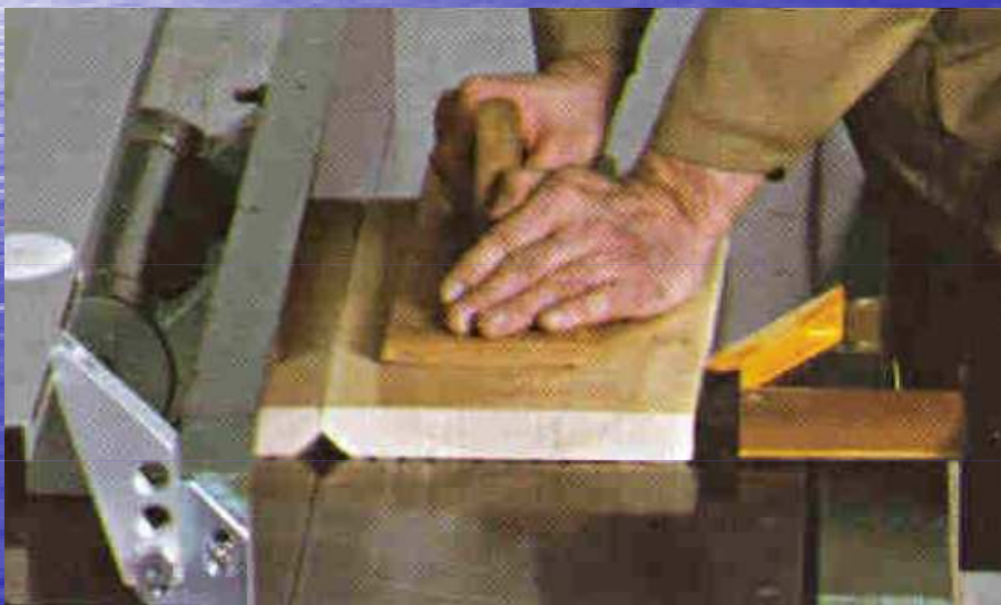
Hoblování dřeva s posouvacím přípravkem
