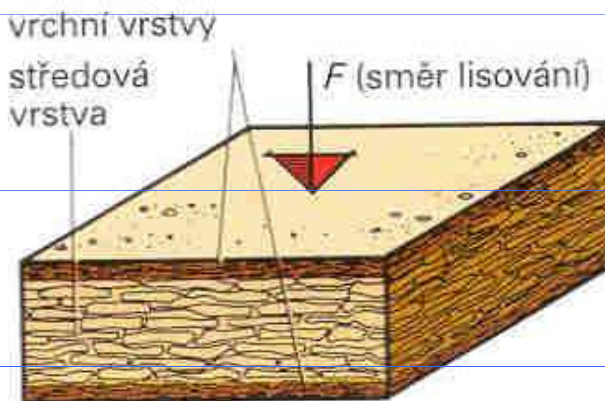
třívrstvá deska
