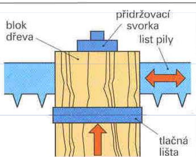
rámová pila na dýhy
