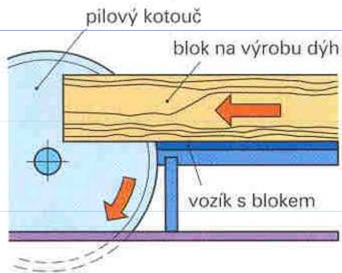
kotoučová pila na dýhy
