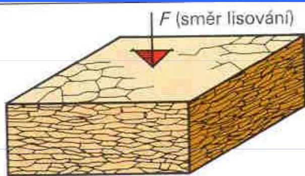
jednovrstvá deska
