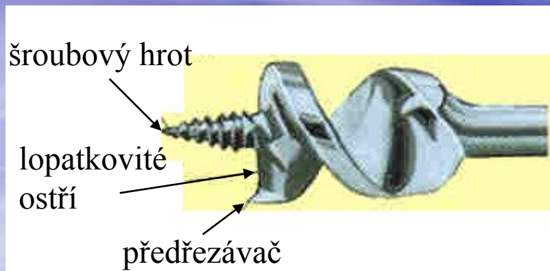
Špulíř
