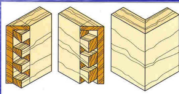
Celokryté ozuby na pokos
