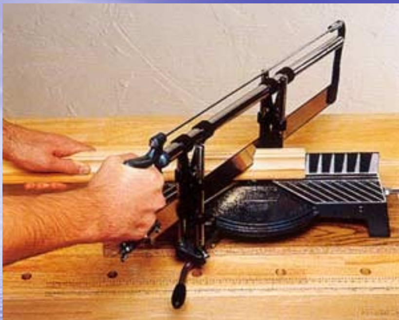
Řezání s pokosovou pilou
