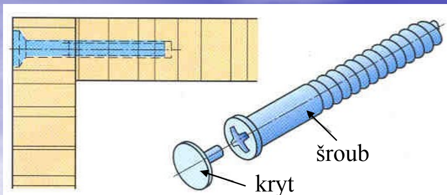
Jednodílný spojovací šroub (confirmat)
