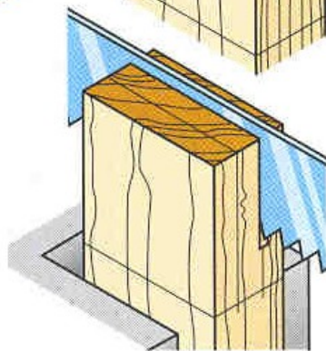
řezání čepu rozporu
