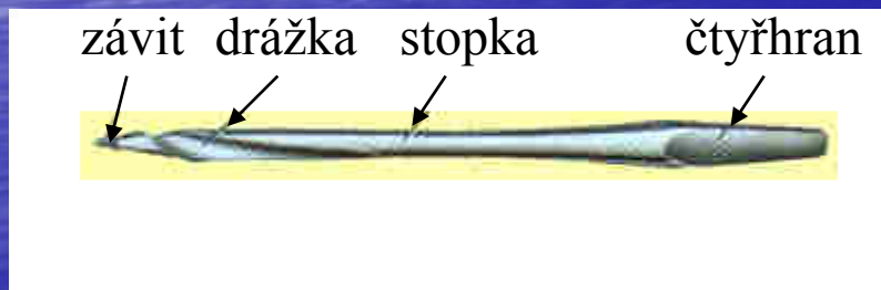
Nebozez s jehlancovou stopkou
