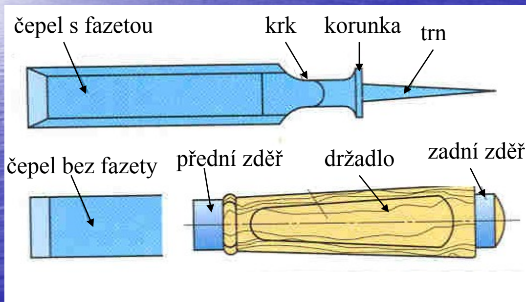
Částí dláta
