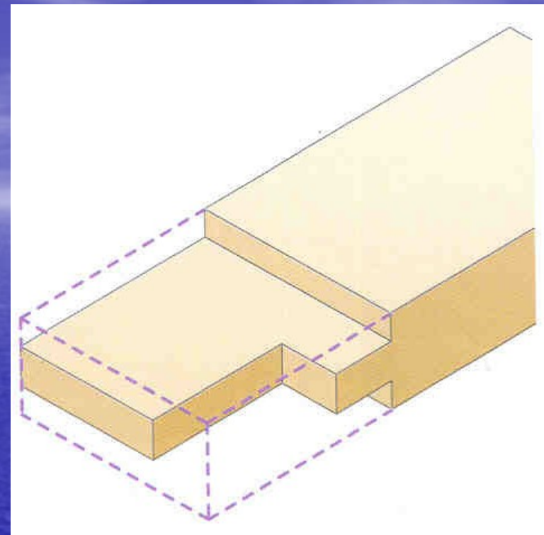
Izometrický náčrt čepu
