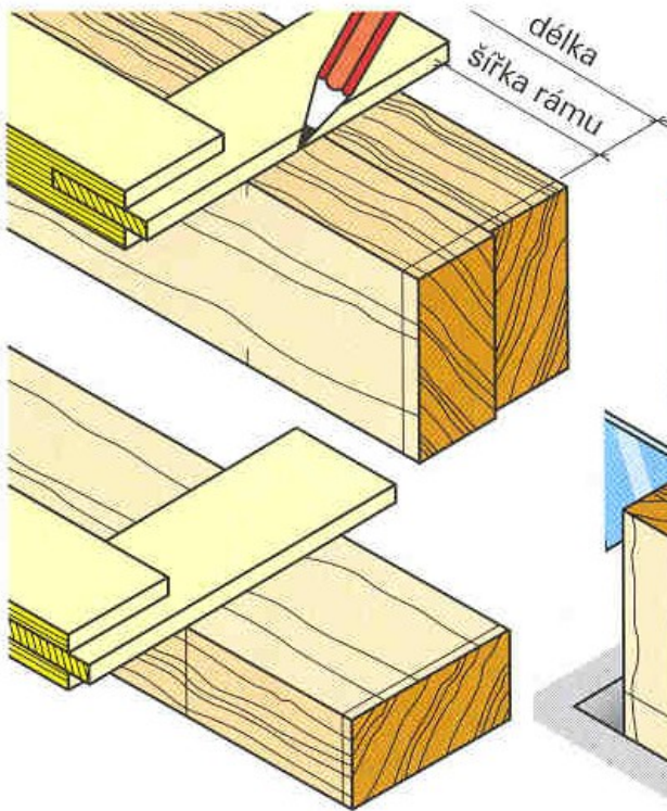
orýsování části s čepem
