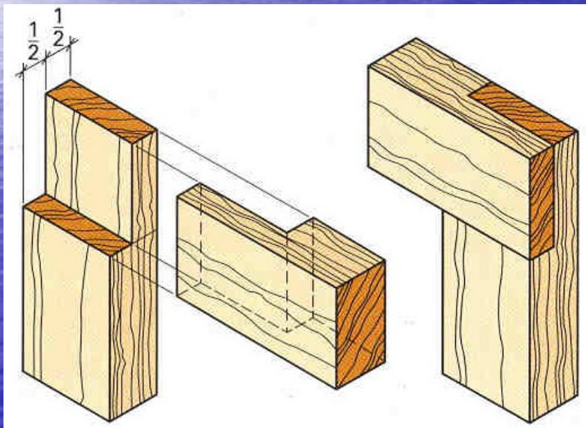
Přeplátování
