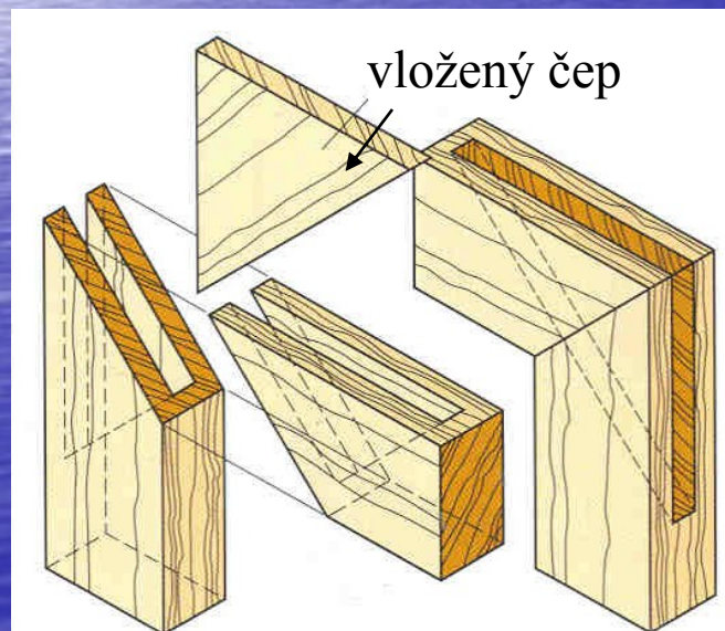
Rohy rámu s vloženým čepem
