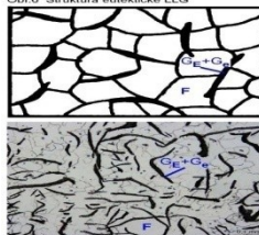
Obr. 6 Struktura eutektické LLG
