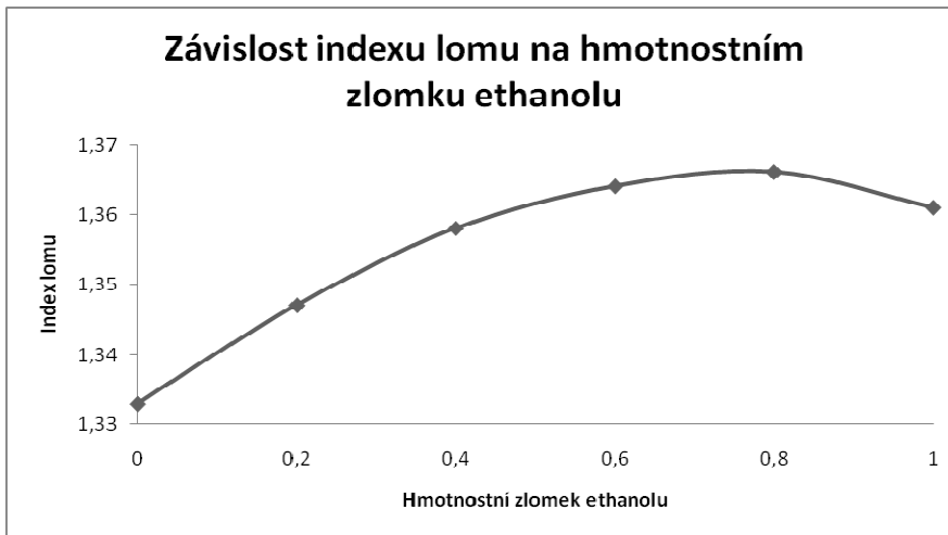
Graf 1: Závislost indexu lomu na hmotnostním zlomku ethanolu.
