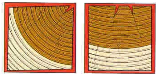
formy sesychání u hranolů
