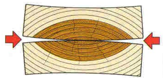
trhání lepených spojů u lepení na tloušťku
