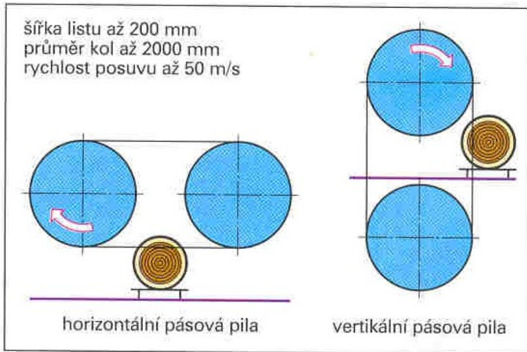
Kmenové pásové pily
