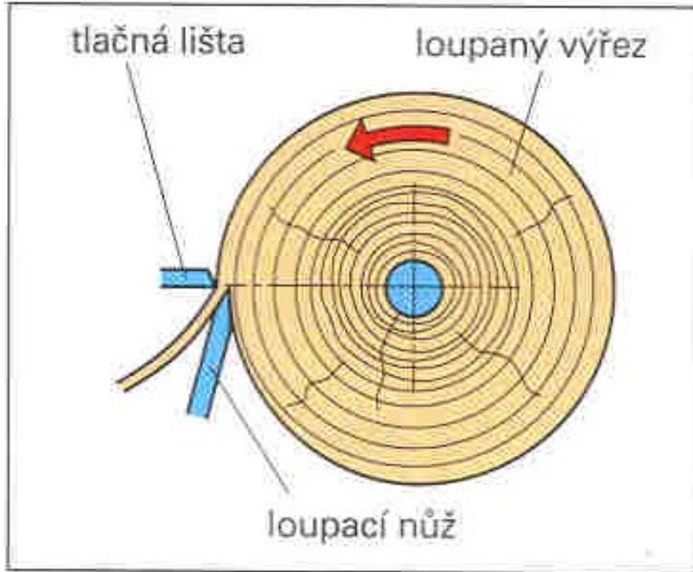
Loupání dýhy (centrické)
