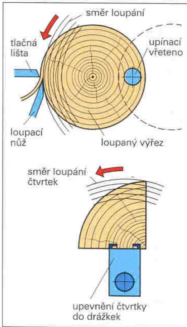
Excentrické loupání dýhy
