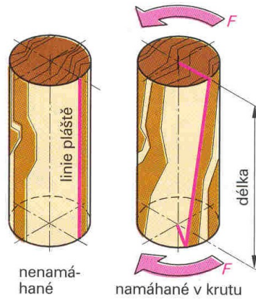
namáhání v krutu
