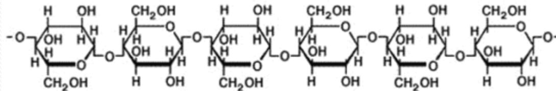
Část molekuly celulózy.
