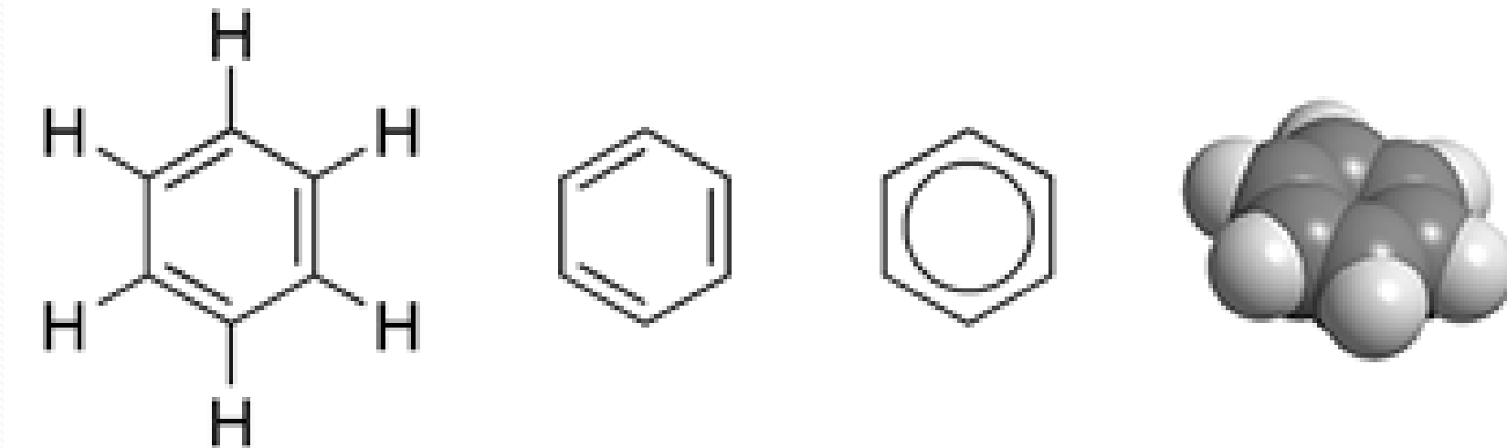
Obr. 1.: Struktura molekuly benzenu
