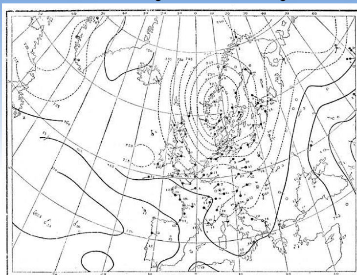
Väderlekskarta på morgonen den 22 oktober 1874.
