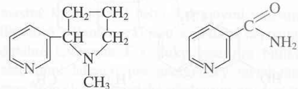
nikotin
