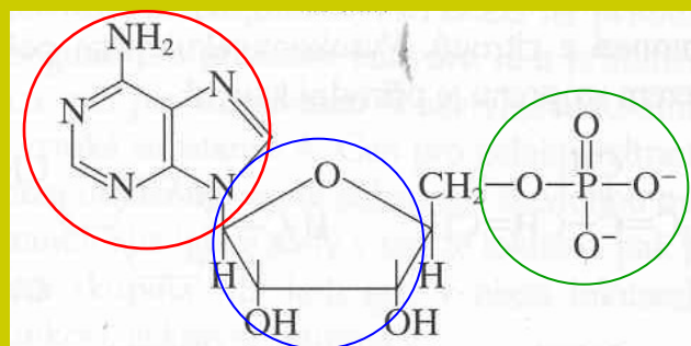
adenin
