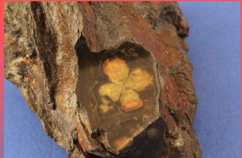
Typický symetrický příčný řez andalusitem – chistolitem v kontaktně metamorfované břidlici.
