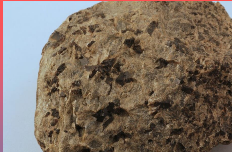
Sloupcovité krystaly staurolitu, některé zdvojčatělé do kříže, svor, Branná.
