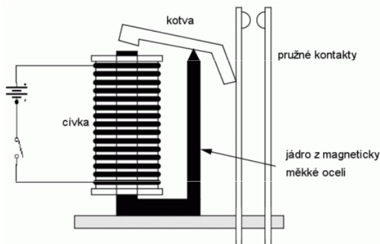
elektromagnetické relé
