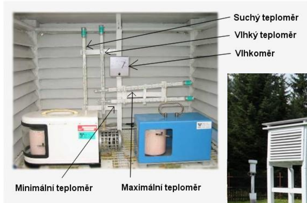
Meteorologická budka
