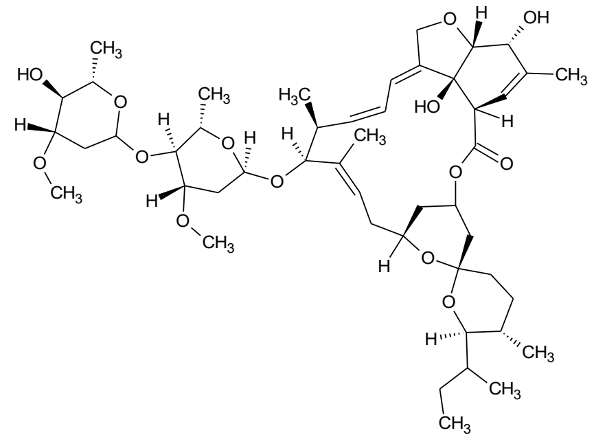
avermektin H2B1b
