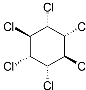
\gamma -hexachlorcyklohexan
