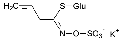
Sinigrin
